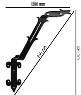
Montagebügel schwarz 55.13.0403
