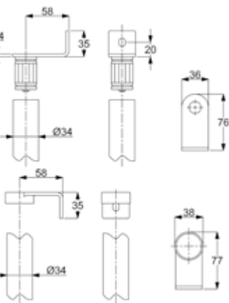
Stoßgriffhalter ohne Befestigungsmaterial, mit Aussenanschluss, für Rohr Ø 33,7 mm
