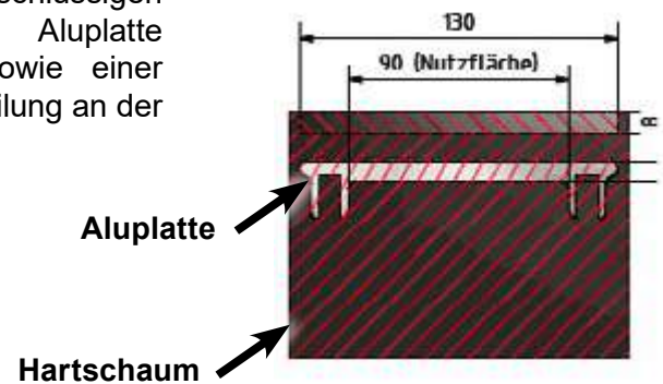
Querschnittzeichnung:
