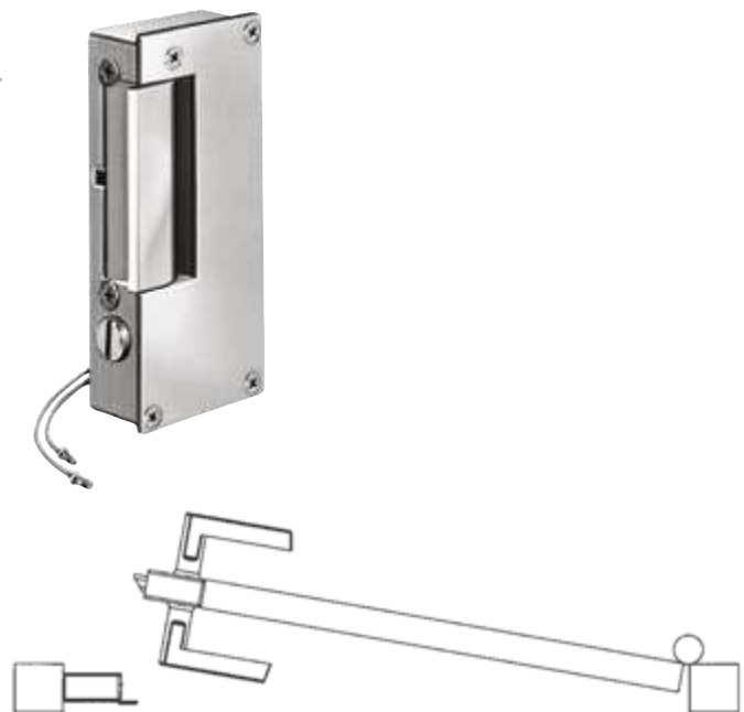
Beispiel: Türanschlag DIN links mit elektrischem Türöffner DIN rechts
