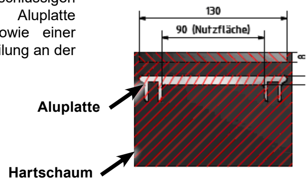
Querschnittzeichnung:
