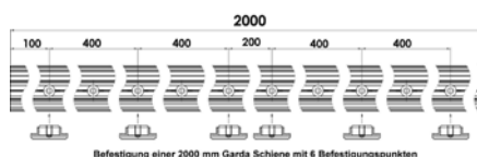
Befestigung einer 2000 mm Garda Schiene mit 6 Befestigungspunkten
